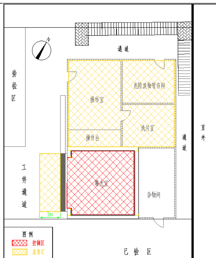
图 10-1 本项目辐射防护两区划分示意图
