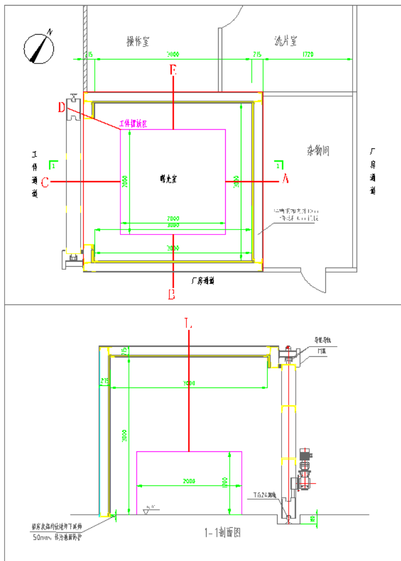
图 11-1 本项目关注点位示意图
