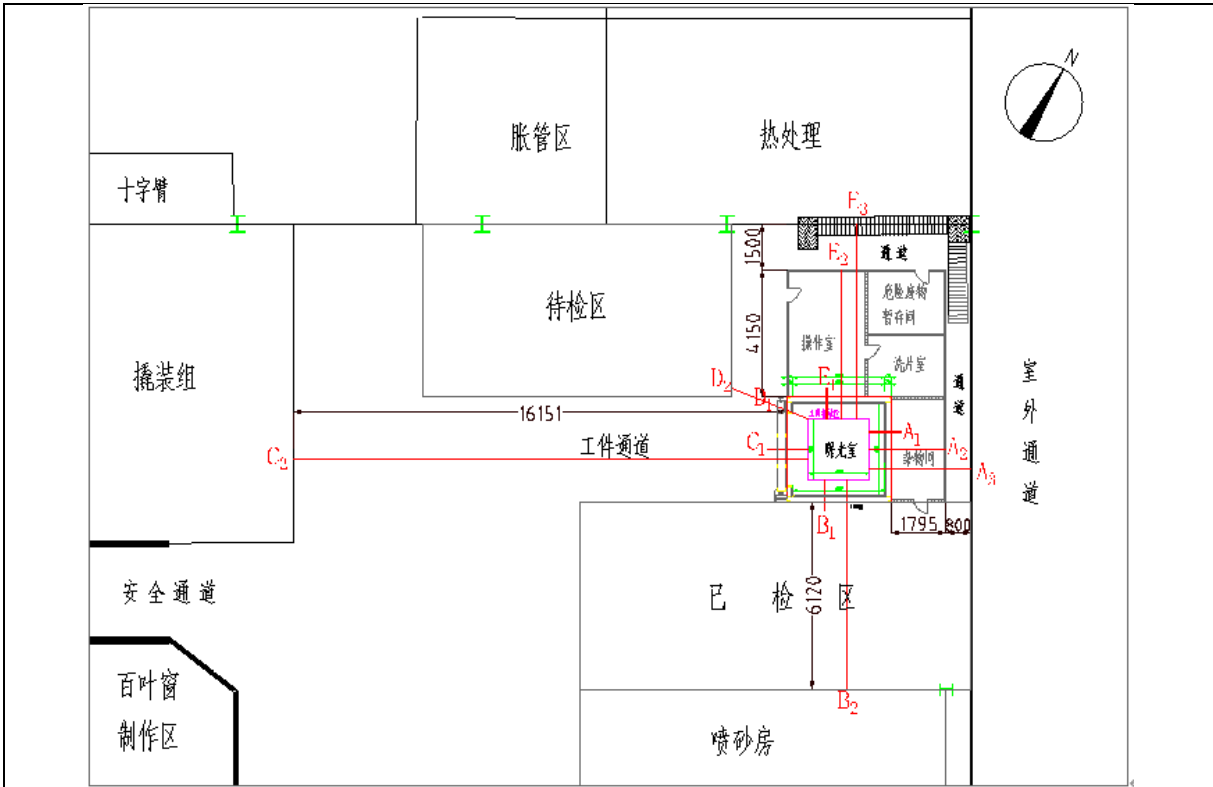
图 11-2 本项目关注点位示意图
